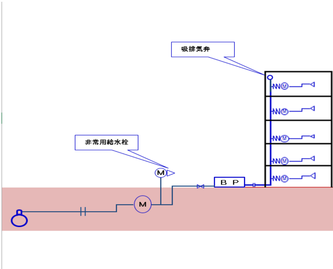
图 5-2 直結增压給水方式(扩大图)
